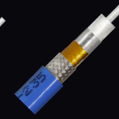
サイズ 235 18 GHz FEP・ETFE被覆 3層編組
