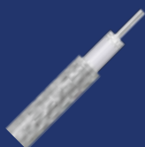
サイズ 047 26.5 GHz 手で曲げ成形可 すず液浸編組
