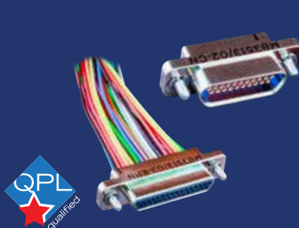
M83513 Micro-D コネクタ・取付金具
