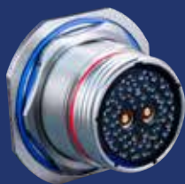
同軸 + 通信 複合配列 ハーメチック
