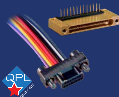
M32139 Nano コネクタ
