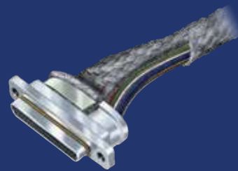
編組シールド付き Micro-Dコネクタケーブルハーネス (カタログ販売)
