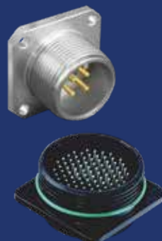
MIL-DTL-5015準拠 ネジ嵌合コネクタ ITシリーズ・ITZシリーズ
