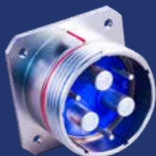
大電流ハーメチック Power-Trip® 最大#1/0コンタクト 定格125A
