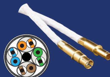
SpeedLine 航空宇宙グレード Glenair El Ochito™ コンタクト 10G Ethernet適合ケーブル
