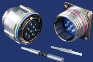
D38999標準 光コネクタ M29504/04・05 光コンタクト
