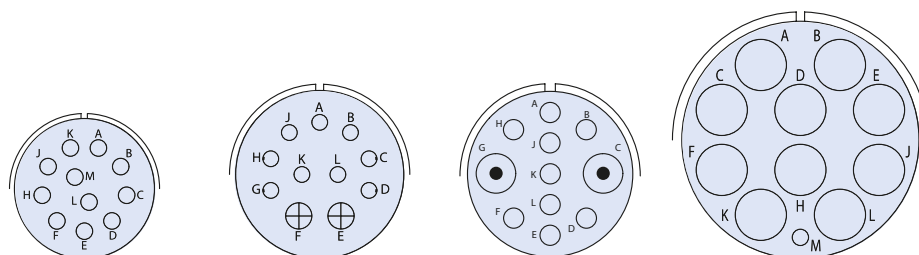
ピンインサートを嵌合面から見た図
