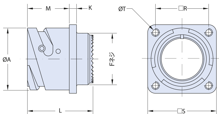
例 : ITS31030A20-27PN0F6 取付穴がスルーホールの場合 例 : ITS31030AFP20-27PN0F6
