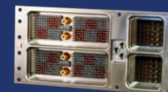
ARINC 600 サイズ1~3 EMIフィルター内蔵
