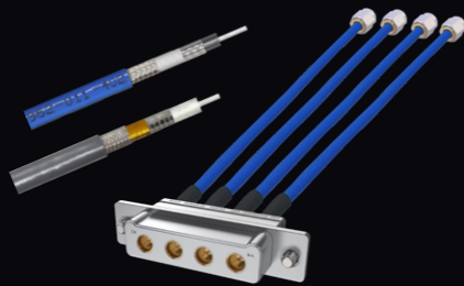
Glenair Dサブコネクタ用 RFコンタクト適合同軸ケーブル
